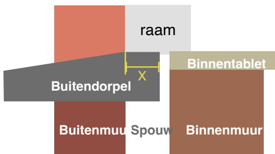
muur met slag (spouwmuur)
