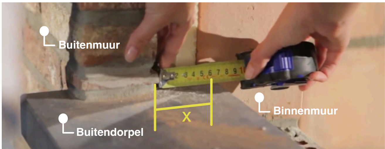
muur met slag (spouwmuur)
